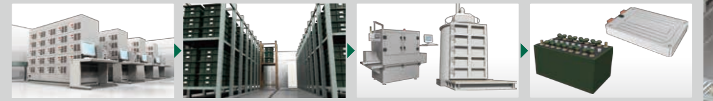
⑳ 充電・放電を繰り返し電池を活性化させます。 ㉑ エージング 満充電の電池セルを所定の温度で一定期間放置します。 ㉒ 検査・スクリーニング 製品としての各種性能を判定します。 ㉓ パッケージング 電池セルを重ねてケースに封入します。
