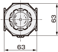
パネルカット寸法 (パネル板厚:MAX.6mm)
