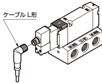
ケーブルL形 (R2)
