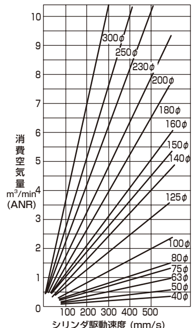
(使用圧力0.5MPa特)
