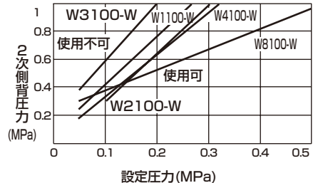
● 背圧に対する設定圧力範囲
