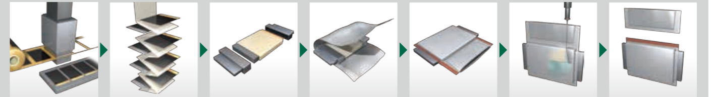
⑦ 電極打抜 正極板・負極板を所定の大きさに型で打ち抜きます。 ⑧ スタッキング 電極とセパレータを交互に高速・高精度で積み重ねます。 ⑨ TAB 溶接 電力を入出力するための接続端子 (TAB) を接合します。 ⑩ ラミネート 電極積層体を外装材で包みます。 ⑪ 熱シーリング 熱を加えセルの3方を接着します。 ⑫ 電解液注液 電池セルに電解液を注入します。 ⑬ ガス抜き・シール 発生したガスを抜きとり、熱を加え電池セルを密封します。
