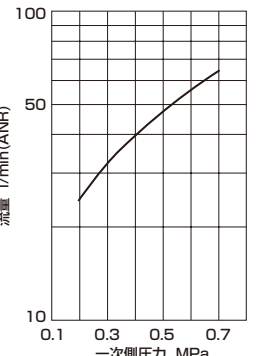
● M1000-W-F1 オートドレン付 (Mタイプ、Sタイプ)
