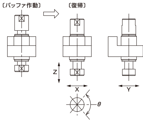
(図1)復帰精度詳細図
