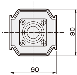
パネルカット寸法 (パネル板厚:MAX.4mm)
